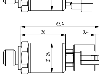
Deutsch DT04-3P
