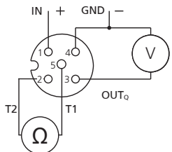
Spannung Ausgang mit PT1000 Voltage output with PT1000 Sortie tension avec PT1000
