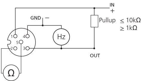
Frequenz Ausgang gefiltert, Impuls Ausgang Frequency output filtered, pulse output Sortie fréquence filtrée, sortie à impulsions
