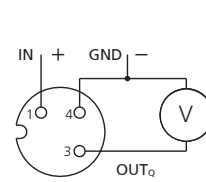
Spannung Ausgang Voltage output Sortie tension
