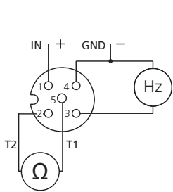
Frequenz Ausgang mit PT1000 Frequency output with PT1000 Sortie fréquence avec PT1000
