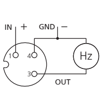
Frequenz Ausgang ungefiltert Frequency output unfiltered Sortie fréquence non filtrée
