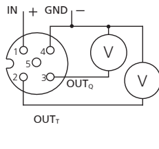
Spannung Ausgang mit 0 ... 10 V Voltage output with 0 ... 10 V Sortie tension avec 0 ... 10 V
