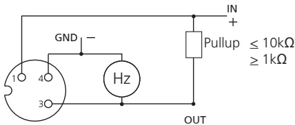
Frequenz Ausgang gefiltert, Impuls Ausgang Frequency output filtered, pulse output Sortie fréquence filtrée, sortie à impulsions
